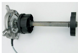
Un pare-chute intégré
