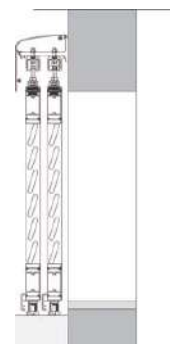
Double voies sur terrasse
