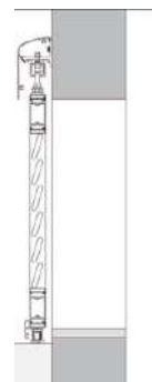
Simple voie sur terrasse
