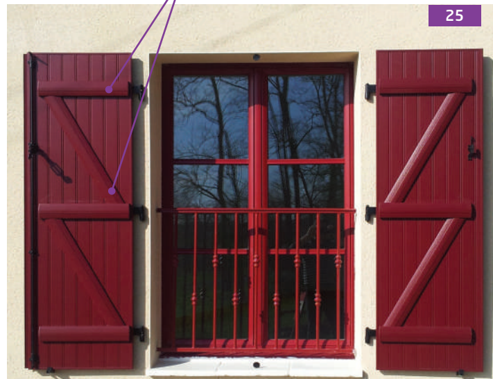
Barres et écharpes
